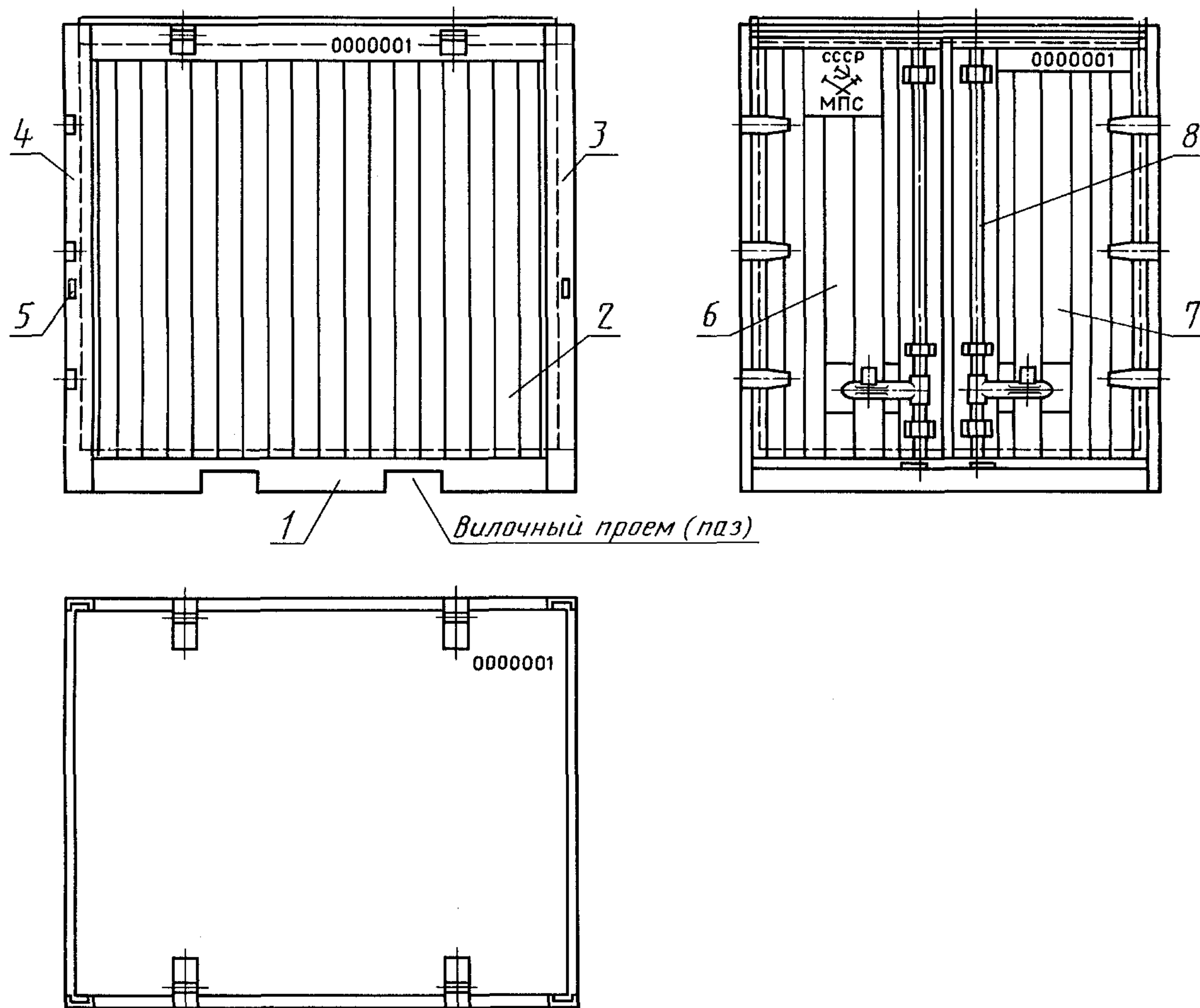
1 — нижняя рама (основание); 2 — боковая стенка; 3 — торцевая рама; 4 — дверная рама; 5 — устройство для крепления контейнера на подвижном составе; 6 — левая створка двери; 7 — правая створка двери; 8 — запорное устройство
